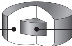
図1 ニフェジピン徐放錠の構造と溶出特性
