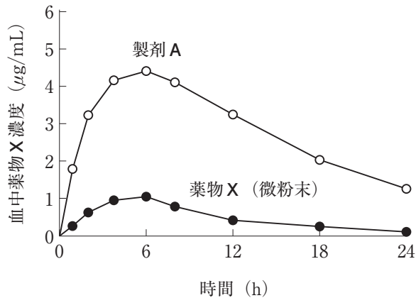
経口投与後の血中薬物濃度の時間推移
