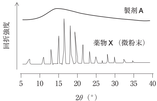
粉末 X 線回折測定の結果
