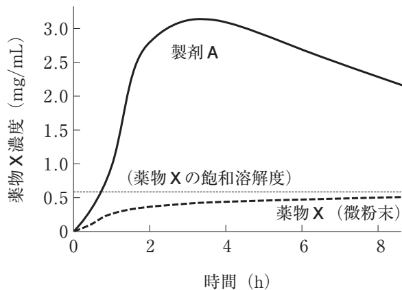
製剤からの薬物の溶出
